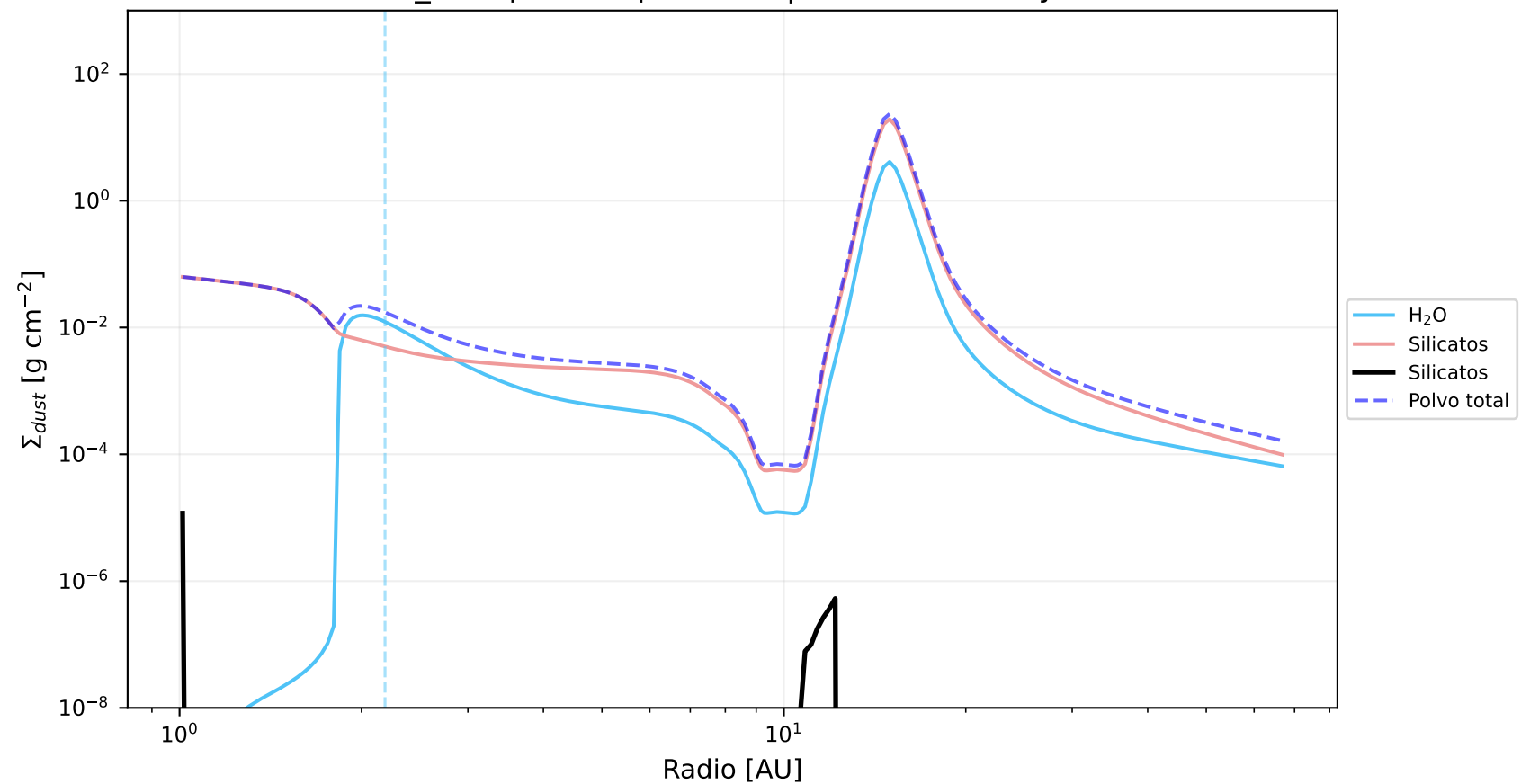
\Sigma_{\text{dust}} por componente | t = 5.00\text{e}+06 yr
